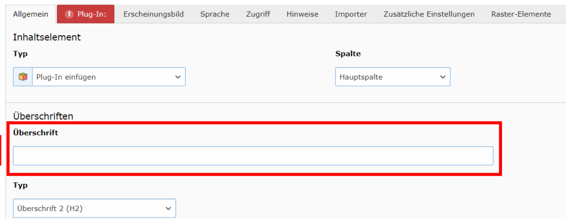
Abbildung 4: Überschrift vergeben
